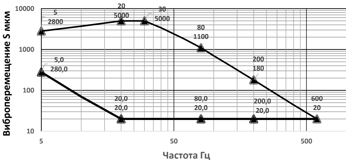
Диапазон измеряемых значений виброперемещения на стенде DVC-500 Bruel&Kjaer 4808
