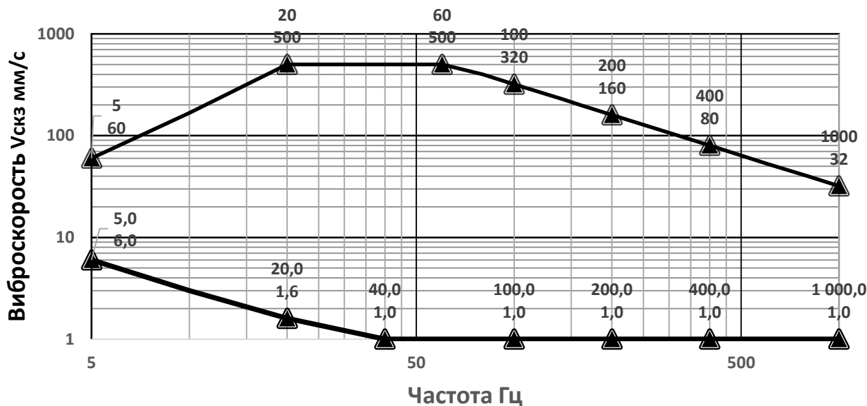
Диапазон измеряемых значений виброскорости на стенде DVC-500 Bruel&Kjaer 4808
