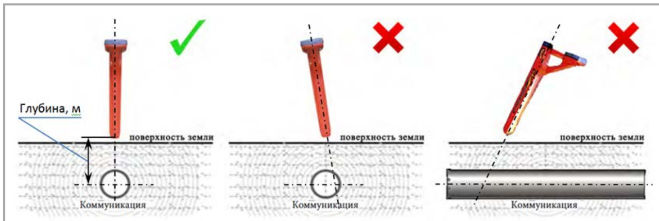
Рисунок 3.6. Правильное положение приемника при замерах глубины.
