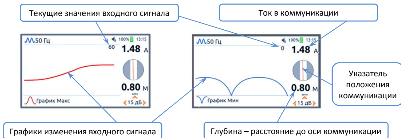
Рисунок 3.13. Режимы «График Макс» и «График Мин».
