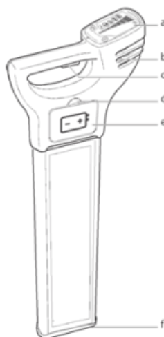
Описание конструкции приемника LKO-1000
