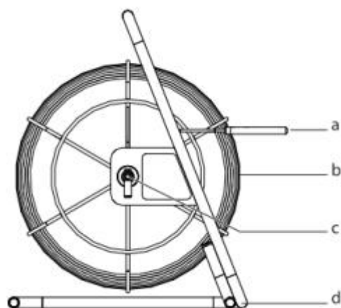
Описание конструкции катушки с локализирующим проводом
