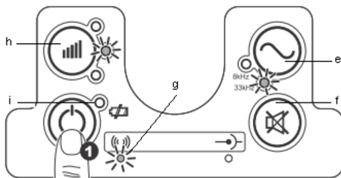
Лицевая панель генератора LKN-1000
