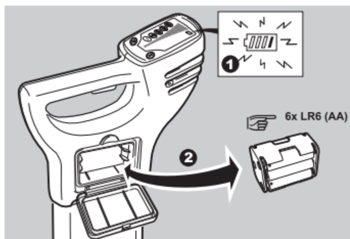
Замена элементов питания в приемнике LKZ-1000
