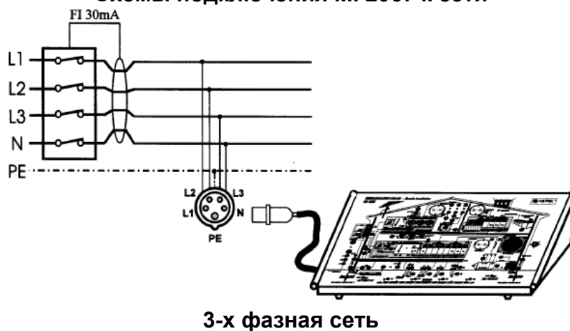
Схемы подключения МІ 2067 к сети
