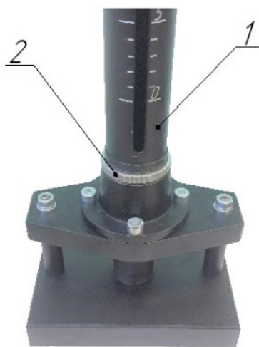
Рисунок 3 – Установка нуля
