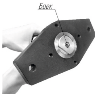
Рисунок 4 – Порядок разборки прибора
