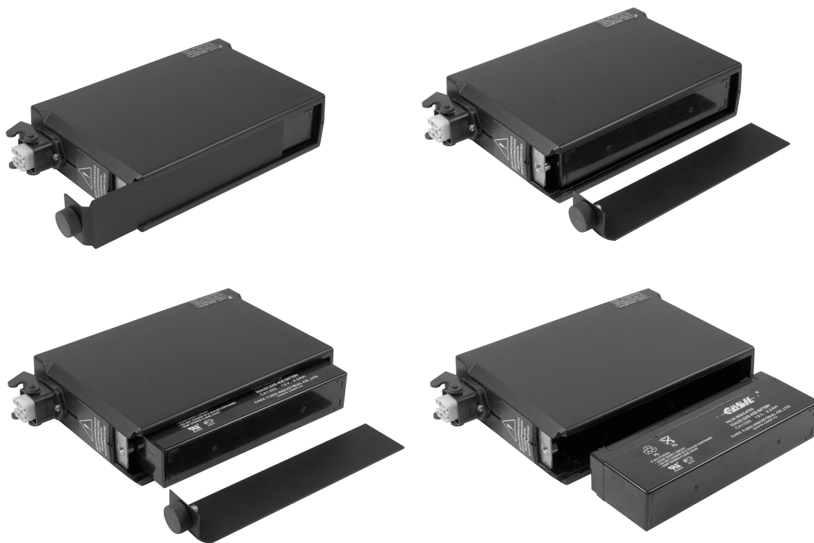
Рис. 31. Последовательность действий при замене аккумулятора
