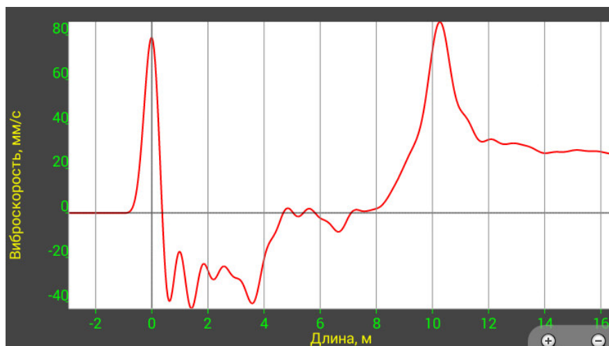
Рисунок 3 – Пример сигнала
